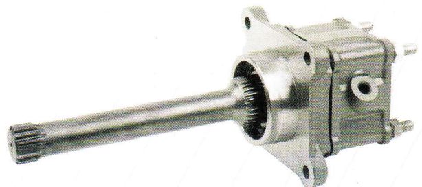
PTO Volvo R 1700 PTO Volvo R 1700
